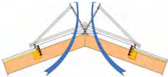
HIWI-First auf Sandwichdach
