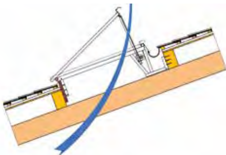
HIWI-Halbe Haube im Dach integriert
